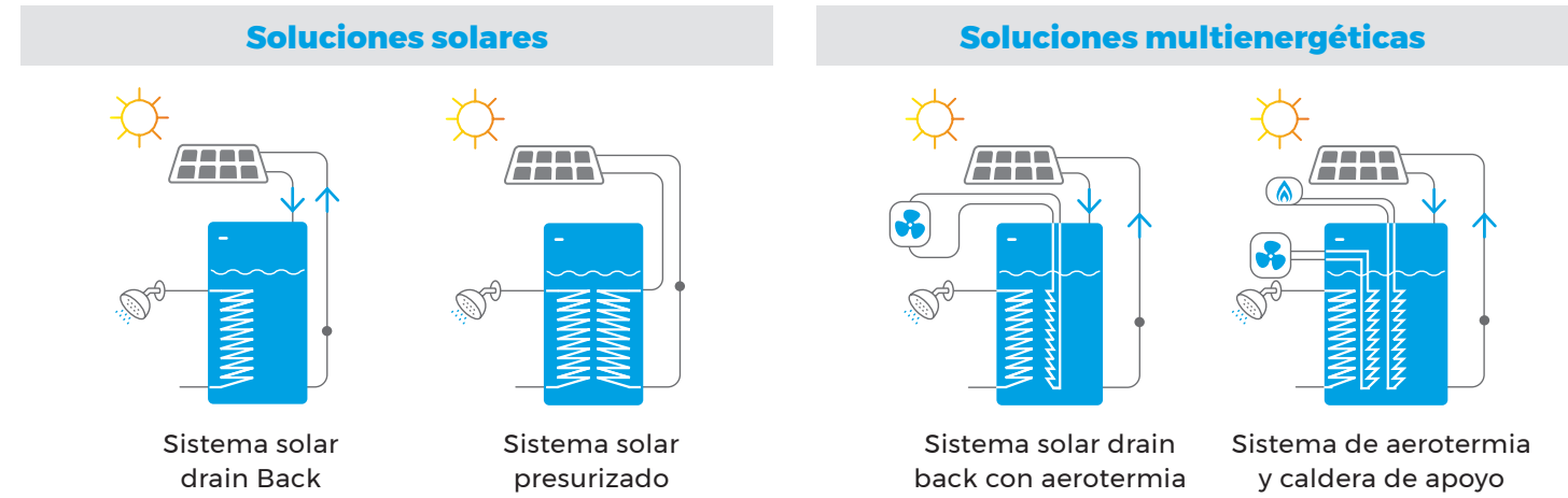
Acumuladores multienergéticos EKHWP-B/PB
