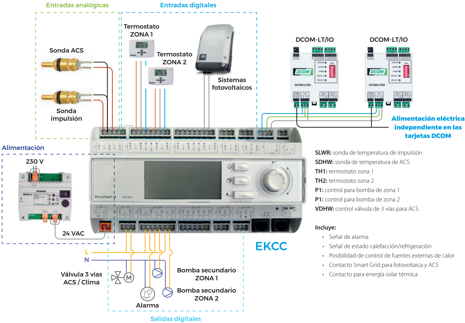
EKCC9-W
