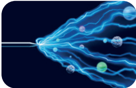
En la descarga de plasma se emiten electrones a alta velocidad
