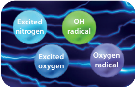
Los electrones colisionan y se mezclan con el nitrógeno y el oxígeno del aire para formar cuatro tipos de elementos
